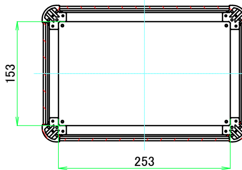
C-C ( 1 : 5.5 )
