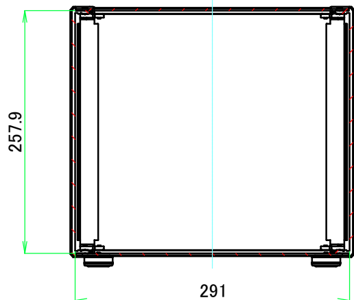
A-A ( 1 : 5.5 )
