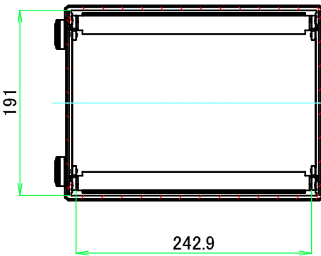
B-B ( 1 : 5.5 )
