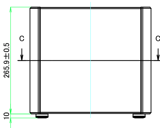
A-A ( 1 : 5.5 )
